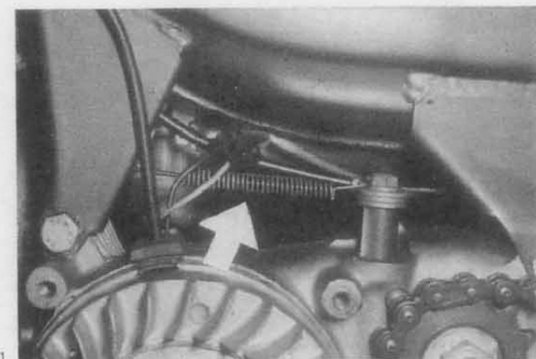
Strom- und Kurzschlußkabel abklemmen. Siehe Bild Nr. 1.
