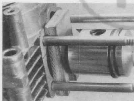
Kolbenholz, Ersatzteil Nr. 09.30.30
