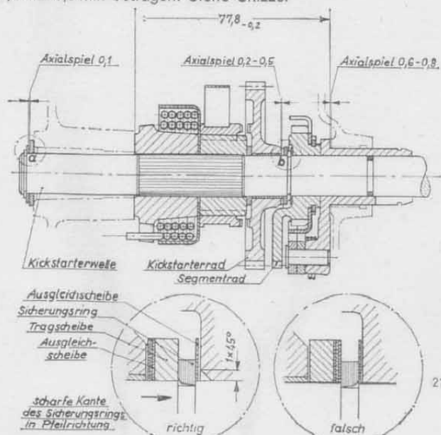
Einzelheit b
