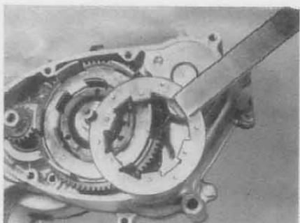
Anhalteschlüssel, Ersatzteil Nr. 09.30.31
